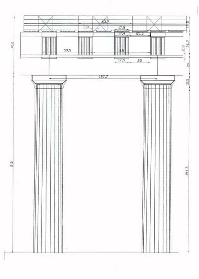
Εικ.2: σχεδιαστική αποτύπωση των δύο κίωνων του προσκηπίου
