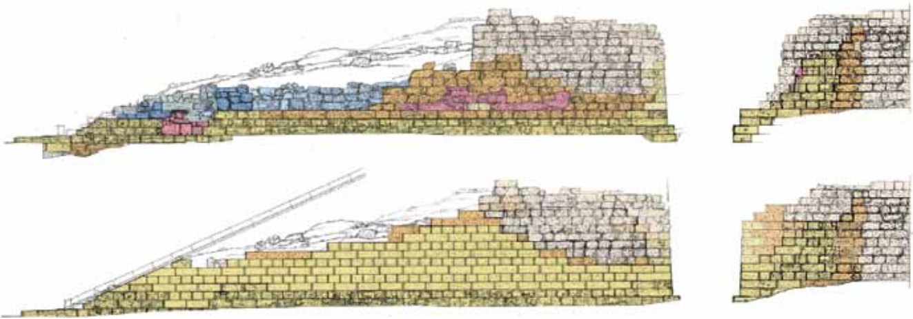
Όψεις του αναλήμματος της ανατολικής παρόδου. Σχέδια αποτύπωσης (επάνω) και πρότασης αναστήλωσης (κάτω).
