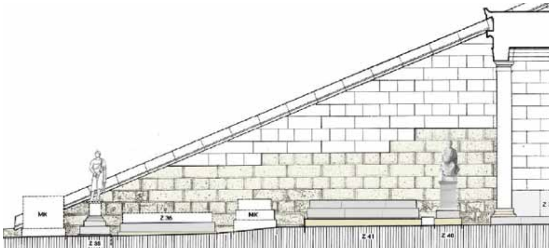
Αναπαράσταση της ανατολικής παρόδου του Θεάτρου. Ο αριθμός Z40 αντιστοιχεί στο άγαλμα του Μενάνδρου.
