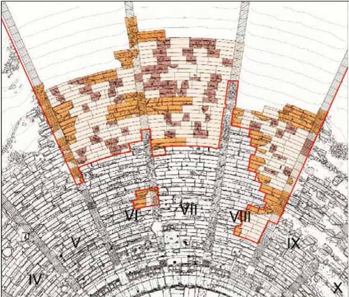
Η εγκεκριμένη πρόταση αποκατάστασης του κεντρικού τομέα Α. Με κίτρινο εικονίζονται οι λίθοι που διατηρούνται στη θέση τους, με καφέ εικονίζονται οι διάσπαρτοι αρχαίοι λίθοι που επανεπεντάσσονται και με υπόλευκο οι νέοι λίθοι.
