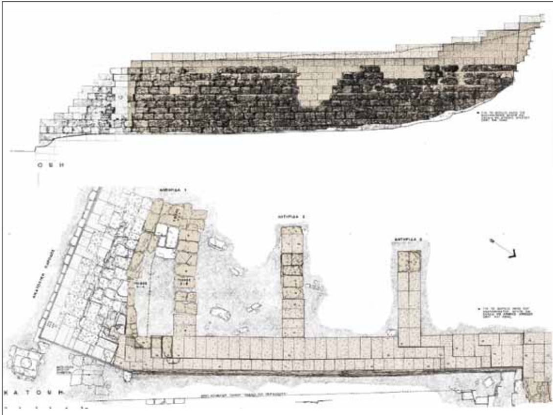
Η εγκεκριμένη πρόταση αποκατάστασης του ανατολικού πλευρικού αναλήμματος
